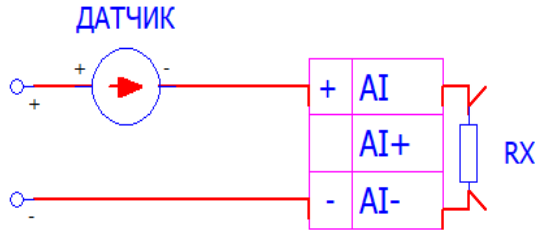
Рис. 3– Схема подключения активного датчика с токовым выходом 0...20 или 4... 20 мА
