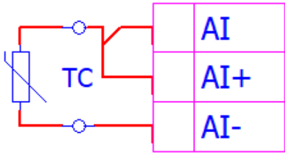
Рис. 2– подключения ТС по трехпроводной схеме
